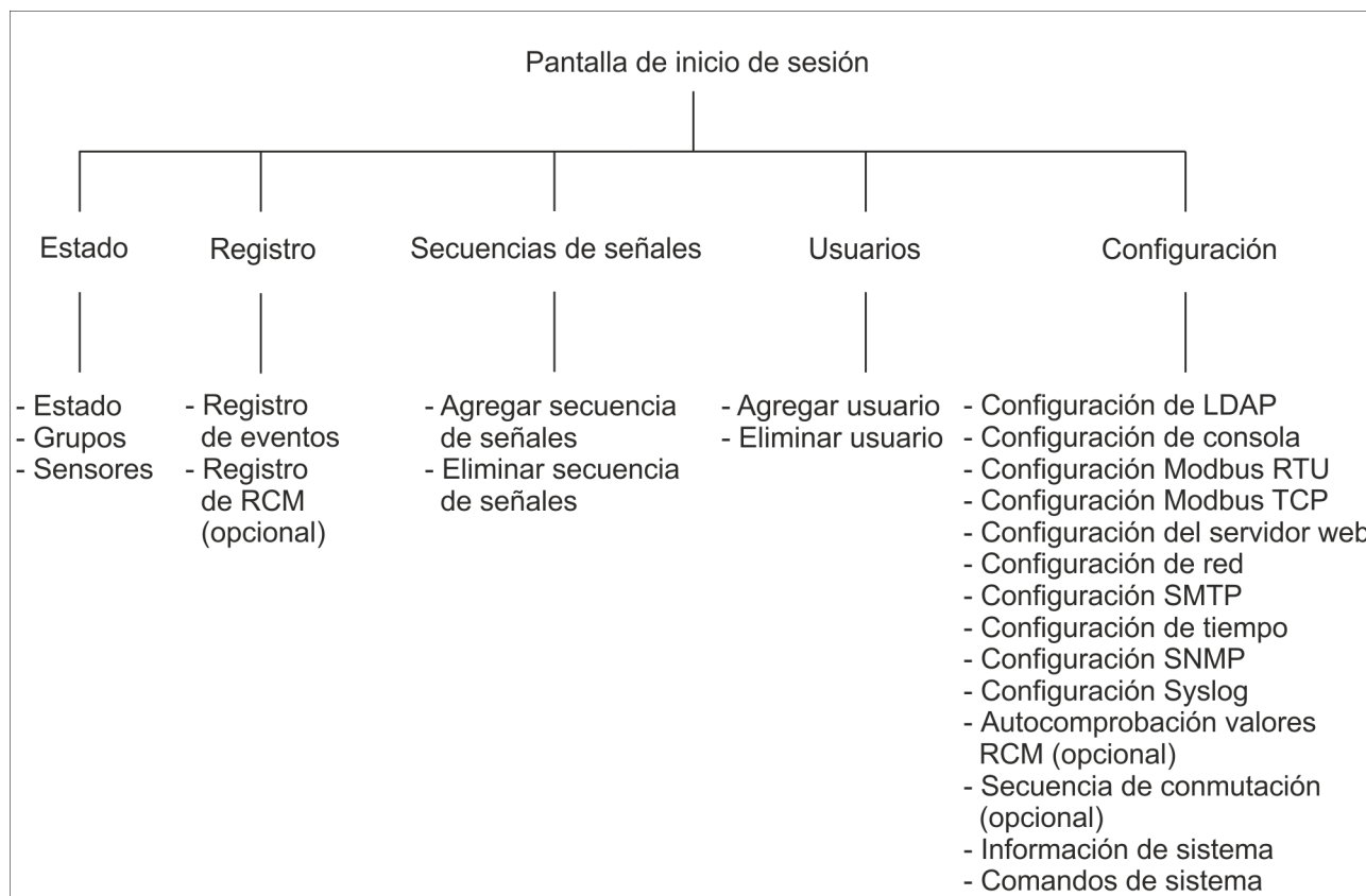
Fig. 86: Estructura del menú de la interfaz web
