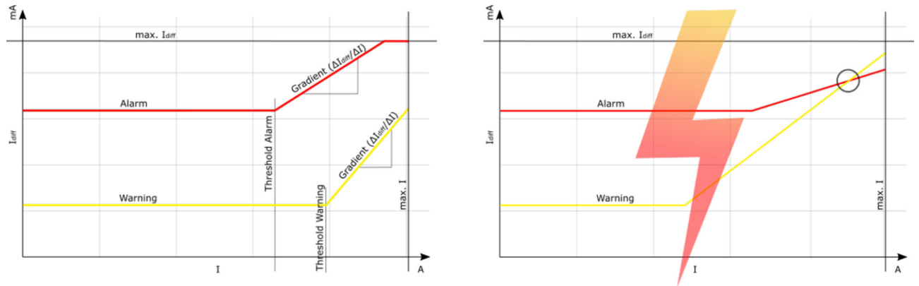
Fig. 18: RCM dinámico
