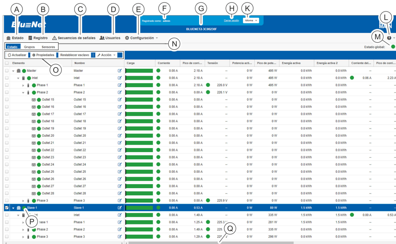
Fig. 89: Vista general de la interfaz web
