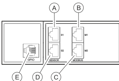
Fig. 4: Zona de conexión (PDU esclava)
