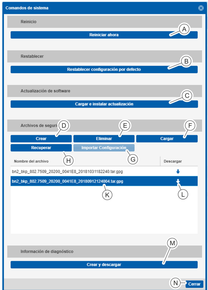
Fig. 145: Ventana "Comandos de sistema"
